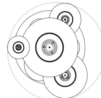
La grappe s'inscrit dans un tube de 850 mm The cluster fits in a tube of diameter 850 mm
