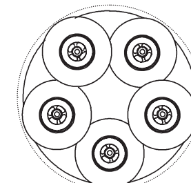
La grappe s'inscrit dans un tube de 260mm The cluster fits in a tube of diameter 260 mm
