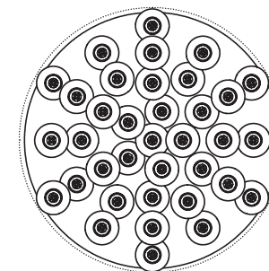
La grappe s'inscrit dans un tube de diamètre 780 mm The cluster fits in a tube of diameter 780 mm
