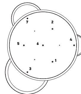
Position des HCS au montage Position of HCS for assembly
