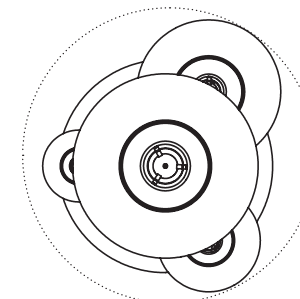
La grappe s'inscrit dans un tube de 770 mm de diamètre The cluster fits in a tube of diameter 770 mm
