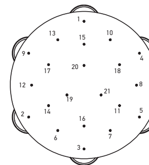
Position des HCS mini au montage Position of HCS mini for assembly
