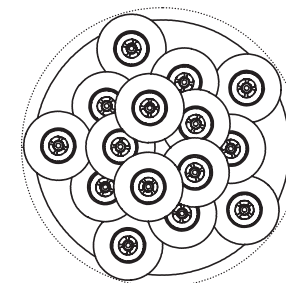
La grappe s'inscrit dans un tube de 400 mm The cluster fits in a tube of diameter 400 mm
