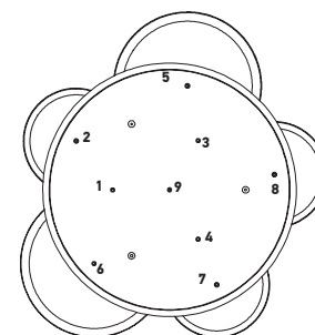
Position des HCS au montage Position of HCS for assembly
