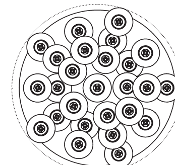
La grappe s'inscrit dans un tube de diamètre 600 mm The cluster fits in a tube of diameter 600 mm
