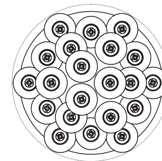
La grappe s'inscrit dans un tube de 490 mm The cluster fits in a tube of diameter 490 mm
