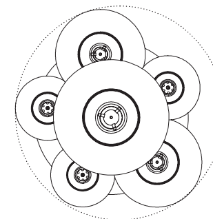
La grappe s'inscrit dans un tube de 1030 mm The cluster fits in a tube of diameter 1030 mm
