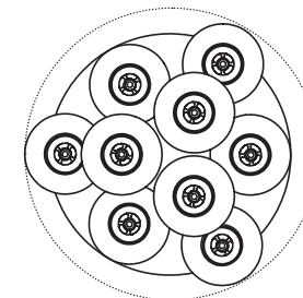
La grappe s'inscrit dans un tube de diamètre 360 mm The cluster fits in a tube of diameter 360 mm
